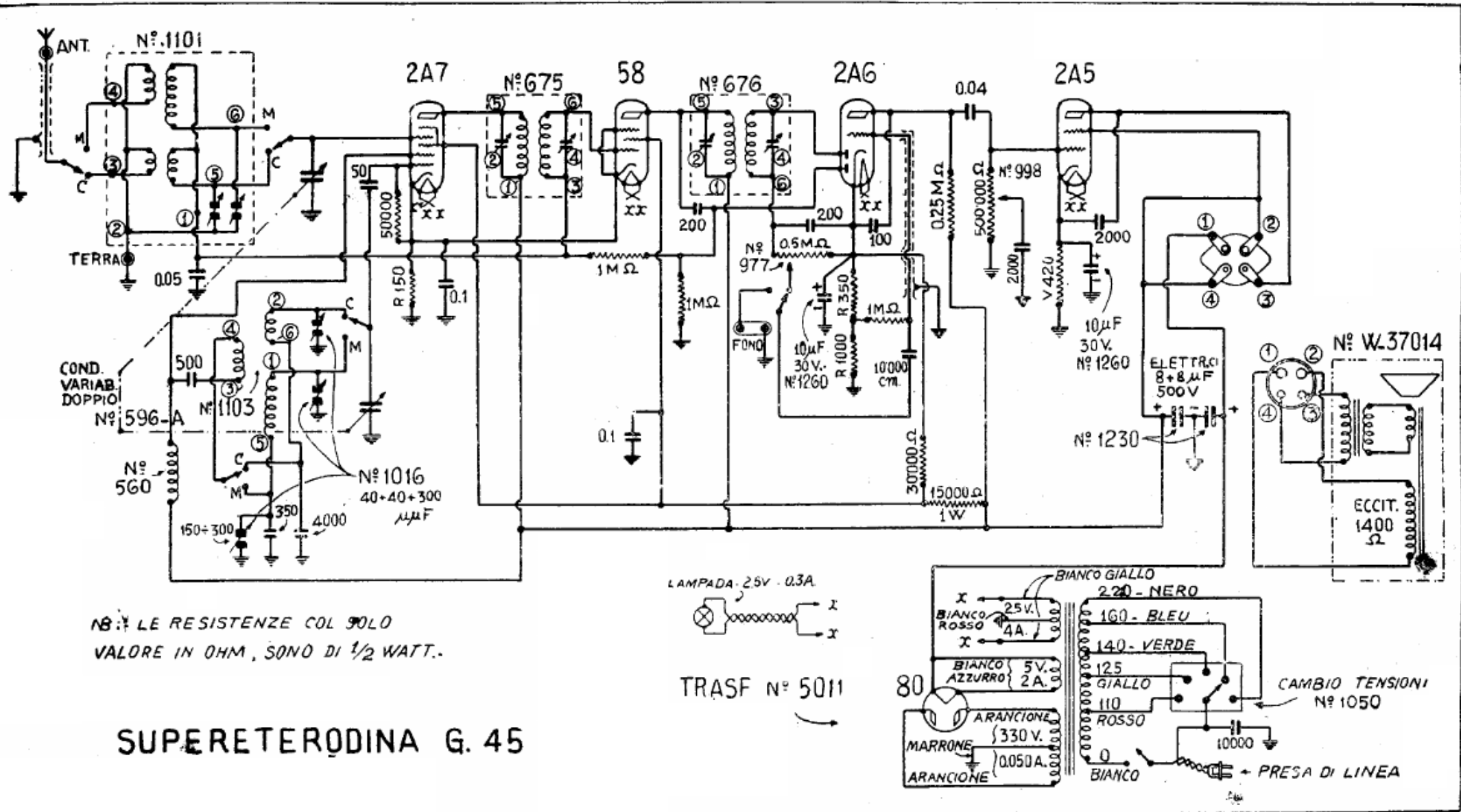
Lo schema elettrico della Super G-45.
